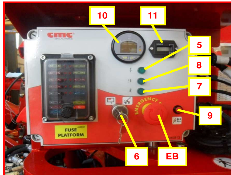
Figure 4b : poste de marche/arrêt du moteur en cas de version hybride ou entièrement au lithium.
